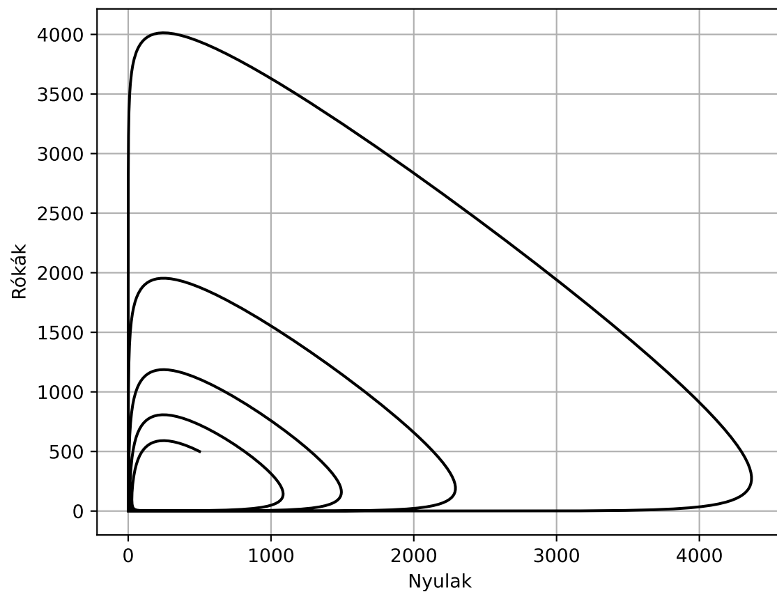
Fázistér
