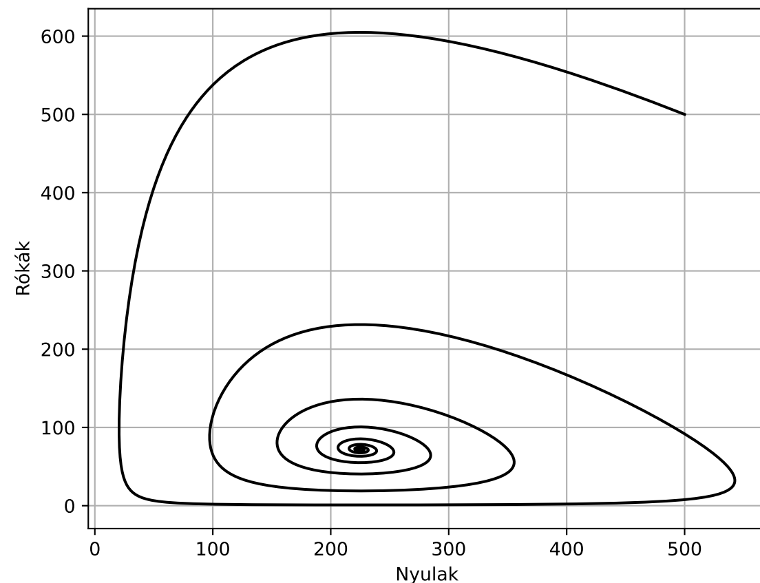
Fázistér
